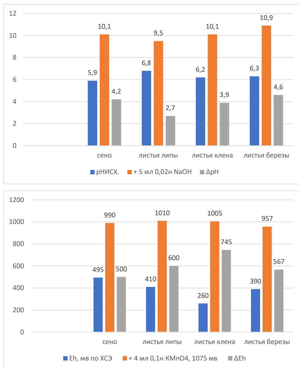
Рисунок 20 – Изменение pH и Eh почвы под действием продуктов разложения растительного опада
