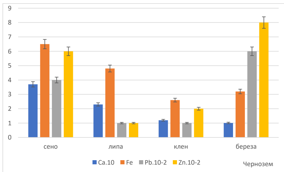
Рисунок 21 – Содержание ионов в почвенных растворах, мг/л
