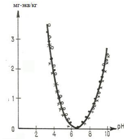
Рисунок 4 – Величина буферности дерново-подзолистой почвы
