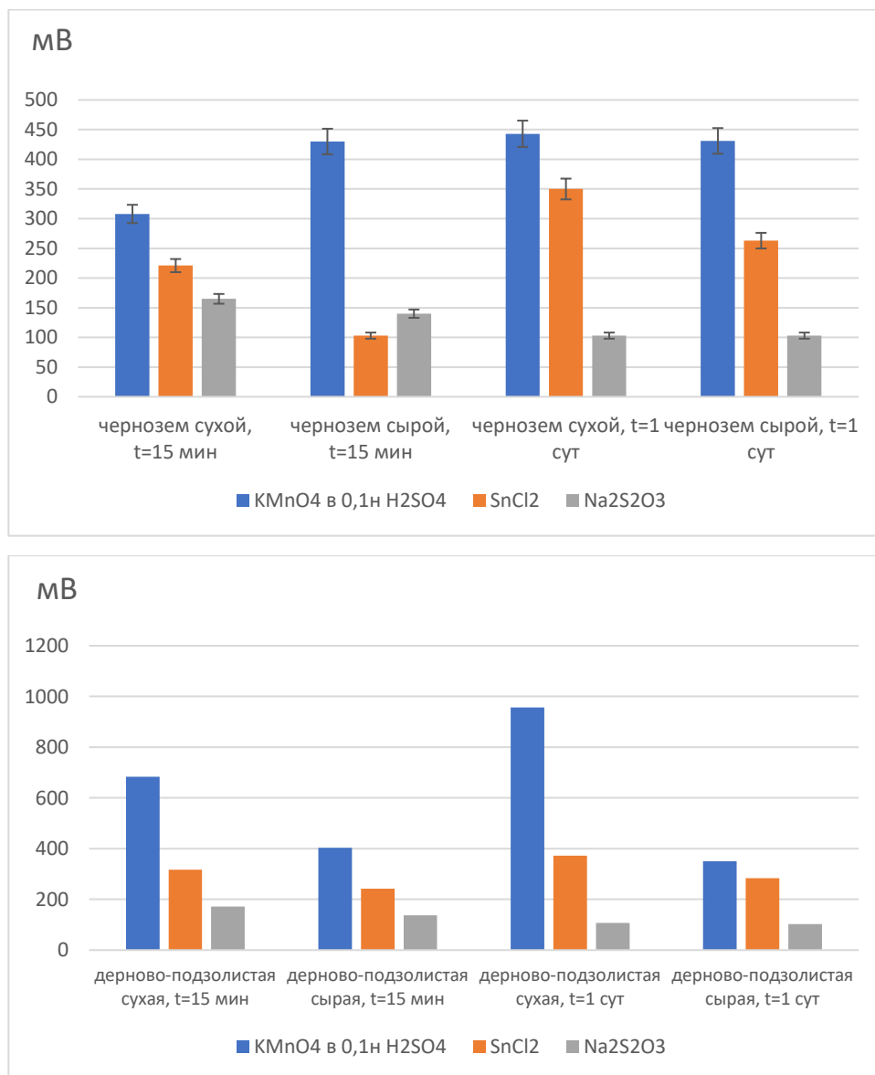
Рисунок 14 - Кинетика окисления и восстановления сухих и избыточно влажных образцов чернозема и дерново-подзолистой почвы
