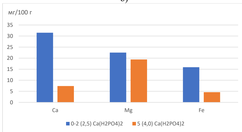
Рисунок 9 - Сумма положительно и отрицательно заряженных соединений Ca, Mg, Fe в зоне внесения удобрений (все почвы), мг/100г (опыт 2)
