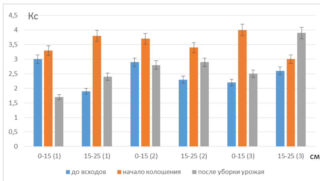
Рисунок 22 - Изменение коэффициента структурности дерново-подзолистой среднесуглинистой почвы в сезонной динамике ( K_c )
