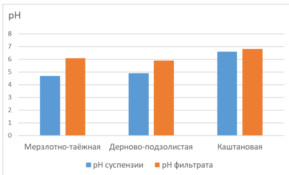
Рисунок 3 - Суспензионный эффект в почвах кислого и щелочного ряда ( pH_{H_2O} )
