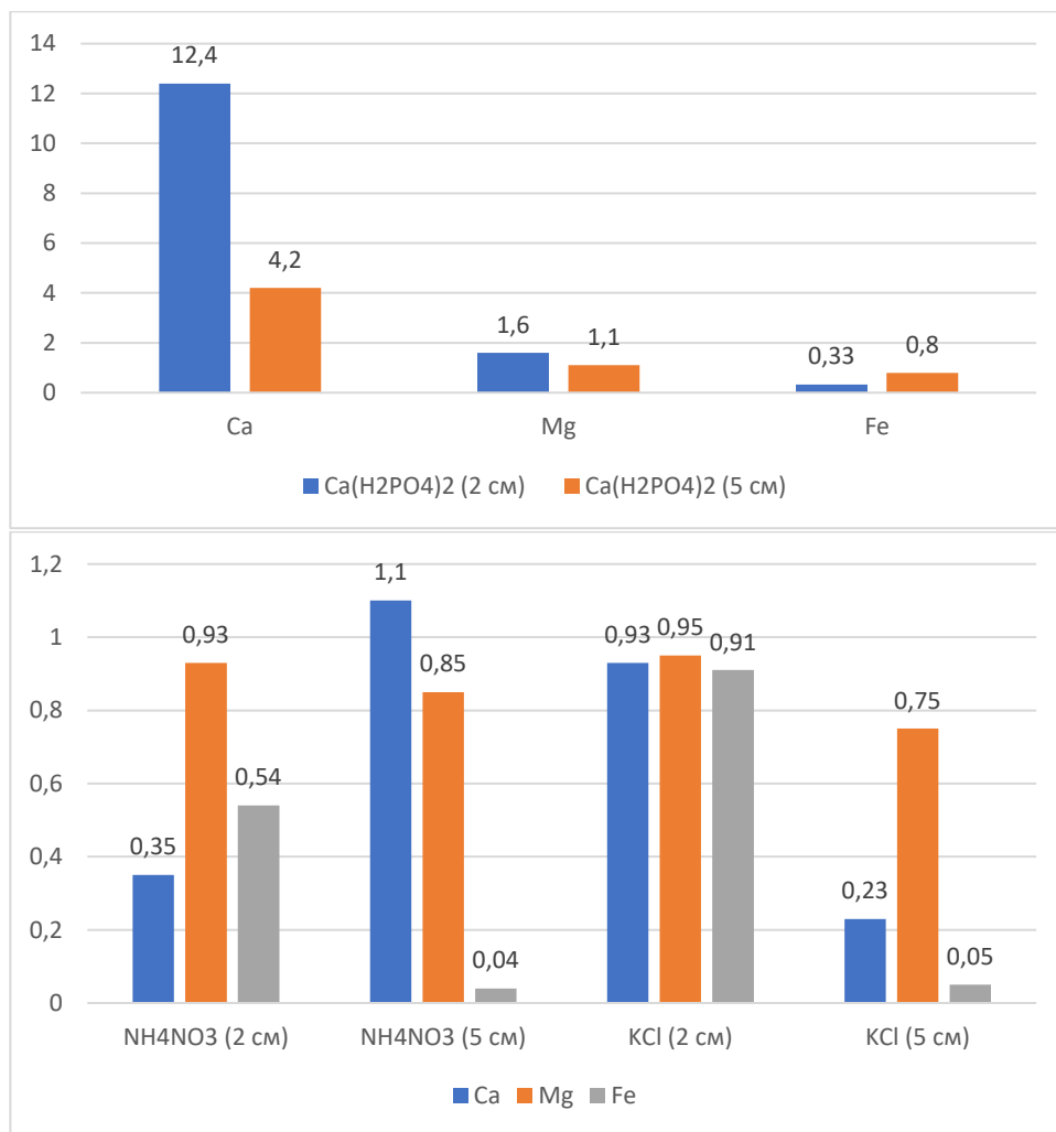
Рисунок 10 - Соотношение положительно и отрицательно заряженных соединений ионов в зоне внесения удобрений, ML^{n+}/ML^{n-}
