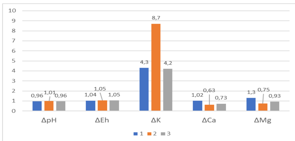
Рисунок 1 - Изменение pH, Eh, концентрации водорастворимых катионов (мг/л) при обработке почвы (An) последовательно возрастающими количествами H_2O (25 и 500 мл)
