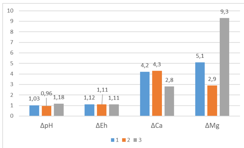
Рисунок 2 - Изменение pH, Eh и концентрации водорастворимых катионов при обработке 0,1н KCl
