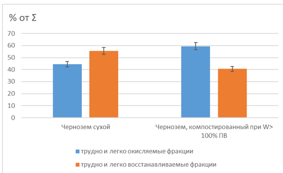
Рисунок 12 - Содержание трудно и легко окисляемых и восстанавливаемых соединений в черноземе (в % от Σ)
