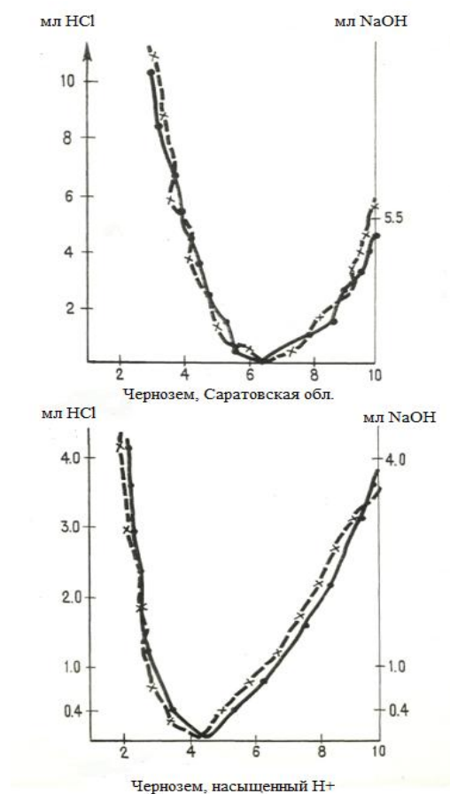
Рисунок 6 - Буферные свойства почв в кислотном и щелочном интервалах
