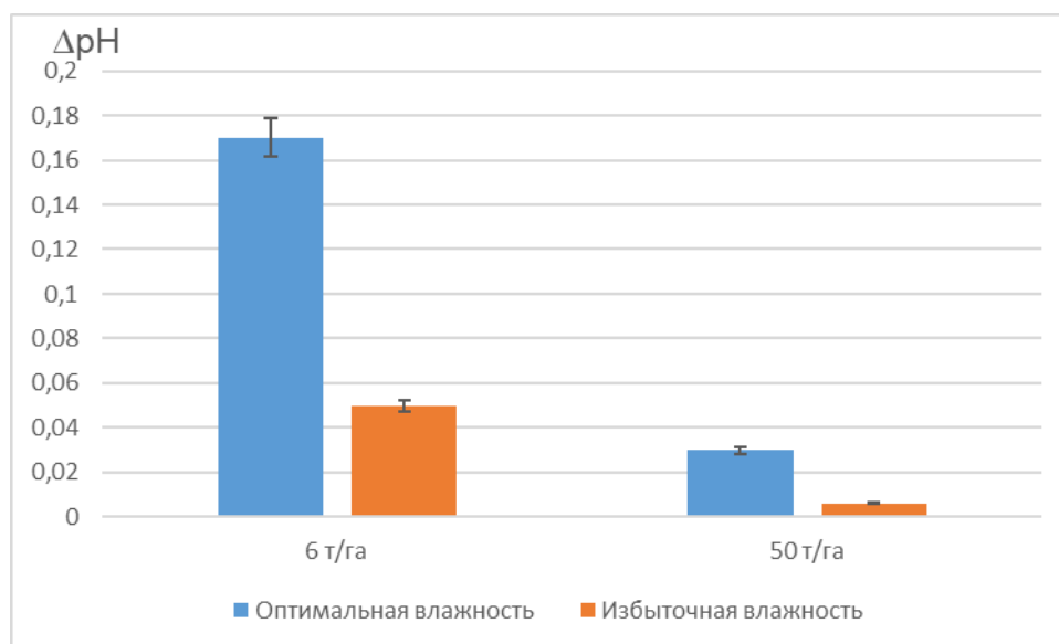
Рисунок 28 - Изменение рН в дерново-подзолистых почвах (площадка 2) при внесении 6 и 50 т/га 1 CaCO 3 (на 1 т CaCO 3 )
