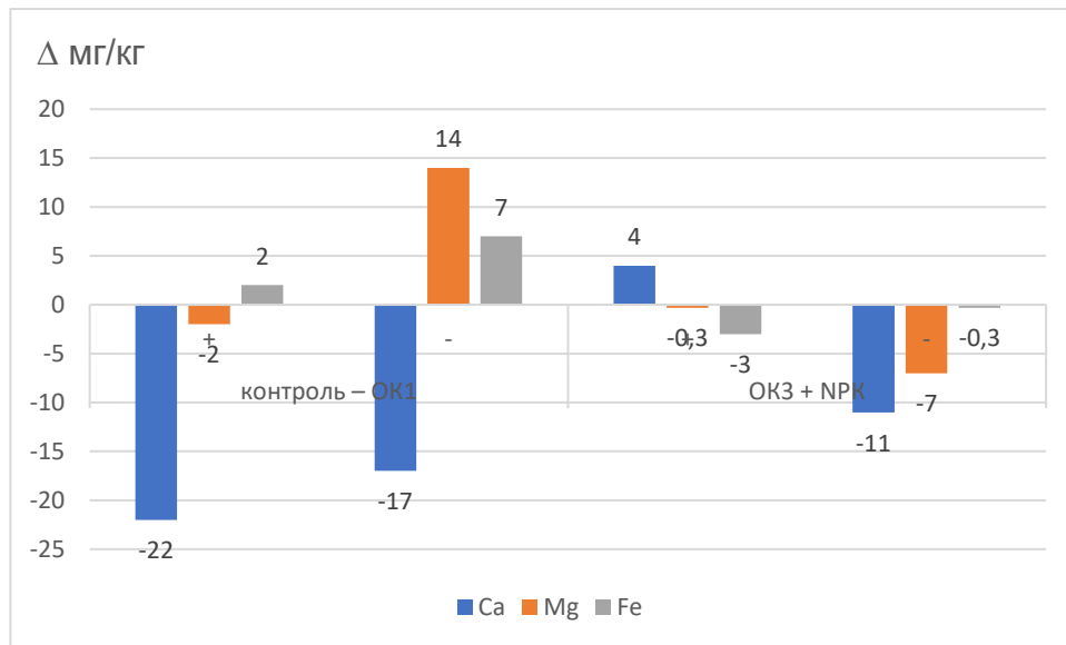
Рисунок 16 - Изменение содержания подвижных элементов в прикорневой зоне дерново-подзолистых почв в зависимости от степени окультуренности почв, Δ мг/кг
