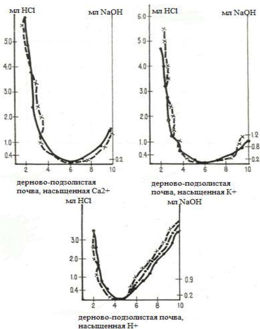
Рисунок 5 – Буферные свойства дерново-подзолистой почвы
