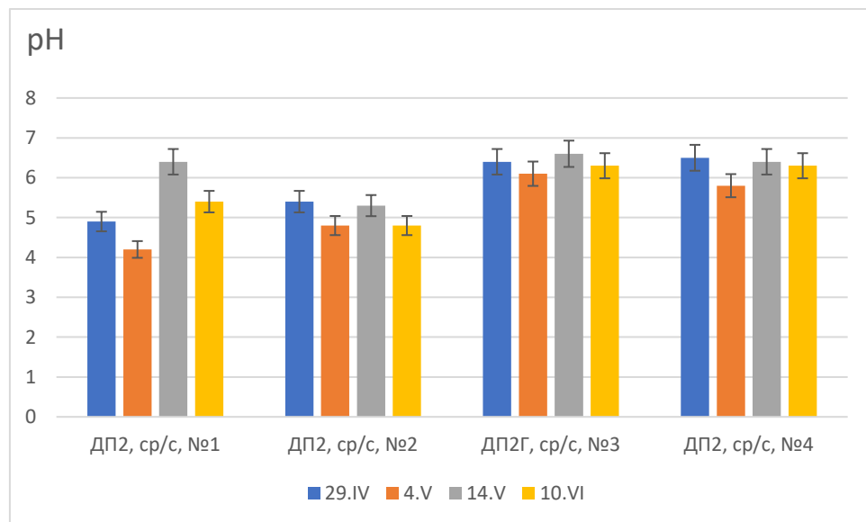
Рисунок 18 - Сезонная динамика изменения pH(H_2O) в дерново-подзолистых почвах разной степени гидроморфности
