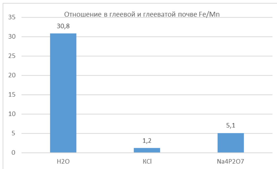
Рисунок 23 – Влияние разной степени гидроморфности в дерново-подзолистых почвах на соотношение Fe/Mn
