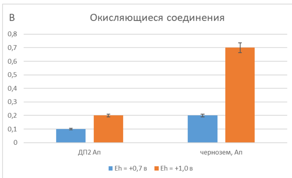
Рисунок 11 - ОВ емкость дерново-подзолистой почвы и чернозема
