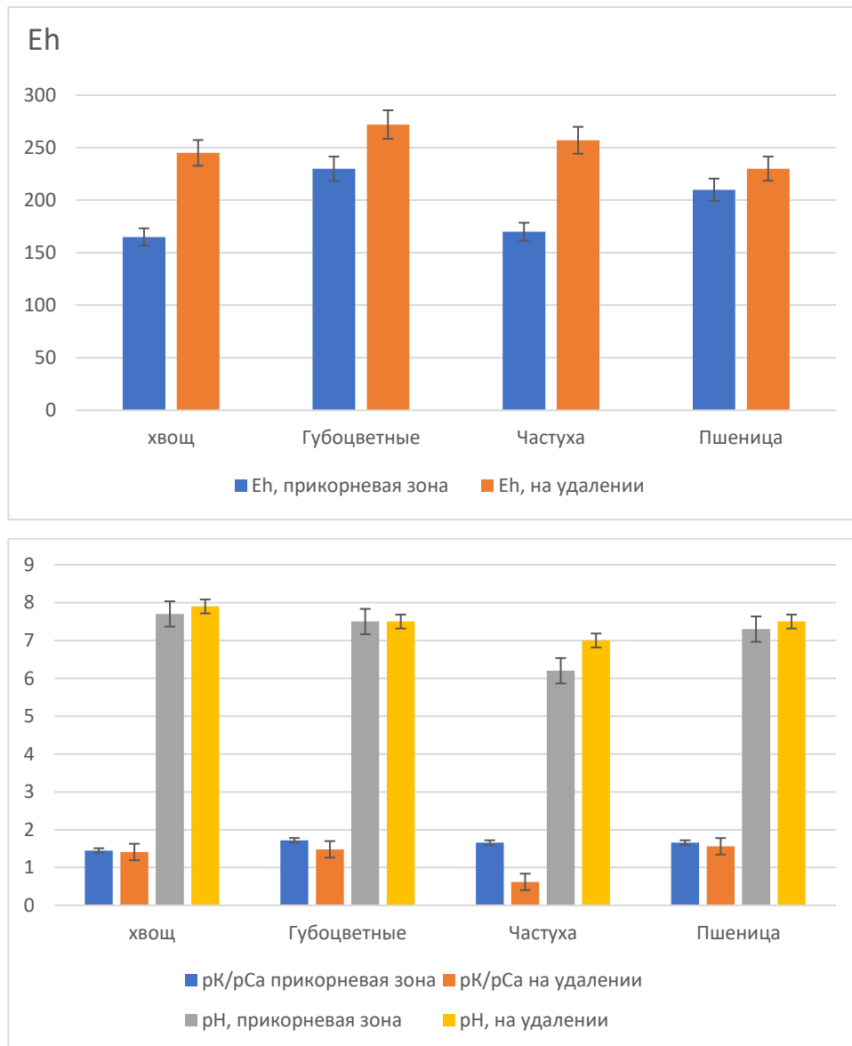
Рисунок 17 - Изменение pH, Eh, активности ионов в прикорневой зоне дерново-подзолистых оглеенных почв по сравнению с остальной массой почв в условиях избыточного увлажнения (в низине)
