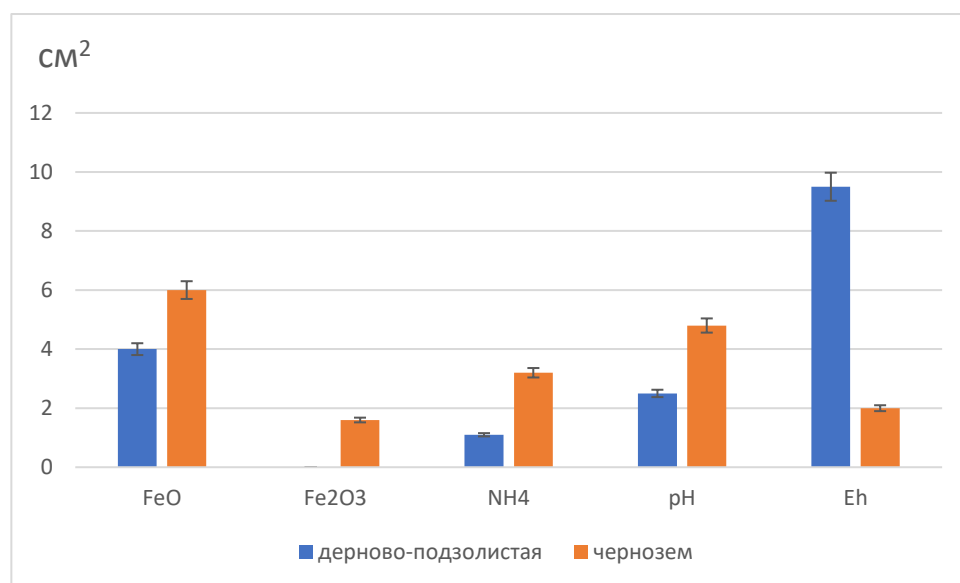
Рисунок 15 - Величина гистерезиса почв по Eh, pH и содержанию подвижных форм железа и азота при смене аэробных и анаэробных условий, см²
