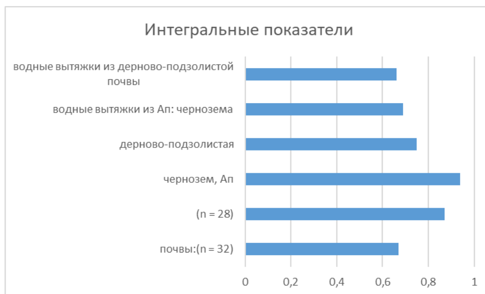
Рисунок 25 - Интегральные энергетические показатели почв и водных вытяжек из них
