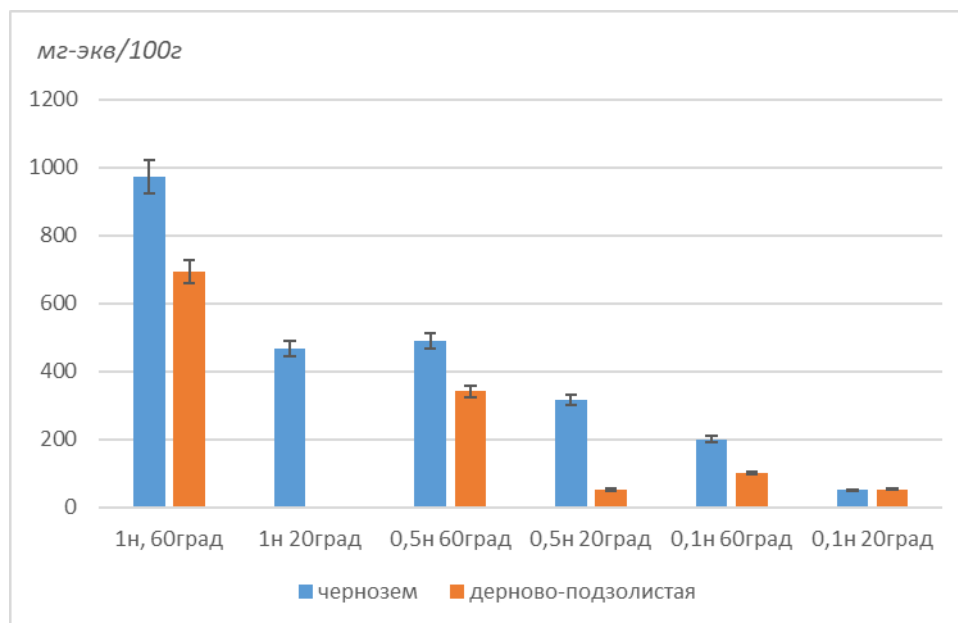
Рисунок 13 - Количество окисляемых KMnO_4 соединений в черноземе и дерново-подзолистой почве, мг-экв/100г
