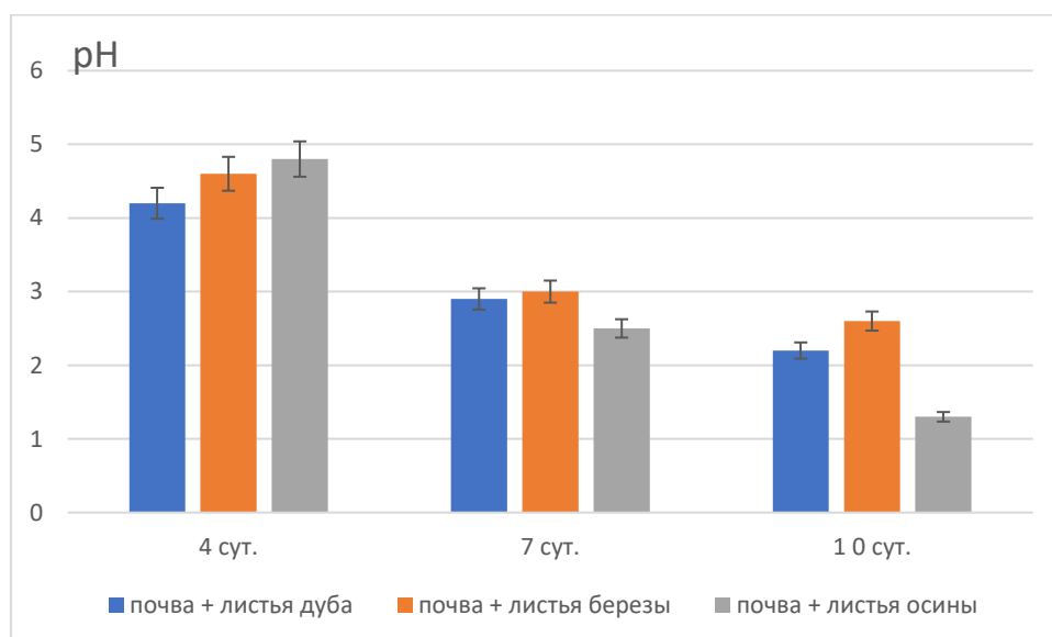
Рисунок 19 - Изменение pH почв при компостировании их с растительными остатками (П:Р = 1:5)
