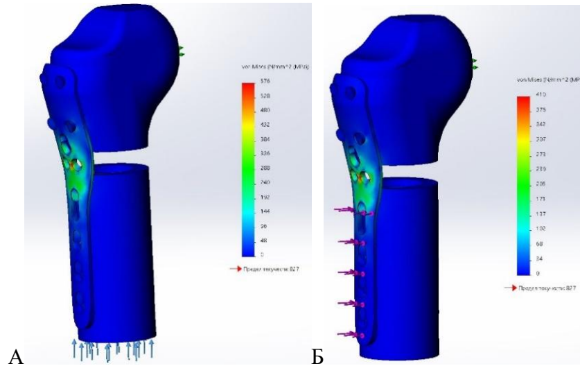
Рисунок 7 – Модель остеосинтеза оскольчатого перелома метафизарной зоны: А – напряжение на деформацию пластины при осевой нагрузке в 300 Н – пластина испытывает напряжения в пределах текучести материала с зонами перегрузок на средней части в области отверстий для винтов, Б – напряжение на деформацию пластины при нагрузках на отведение в плечевом суставе в 100 Н – пластина испытывает напряжения в пределах текучести материала с зонами перегрузок на средней части в области отверстий для винтов
