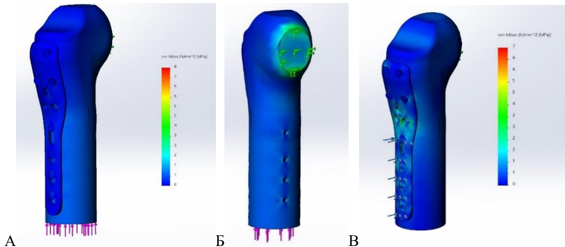
Рисунок 10 – Модель консолидированного в условиях накостного остеосинтеза перелома: А – напряжение на деформацию пластины при осевой нагрузке в 300 Н – пластина не испытывает напряжения, Б – отверстия от винтов в медиальном кортикале плечевой кости испытывают напряжения в пределах текучести, В: напряжение на деформацию пластины при нагрузках на отведение в плечевом суставе в 100 Н – пластина испытывает напряжения в пределах текучести материала с равномерным распределением напряжений преимущественно в центральном и дистальном участках
