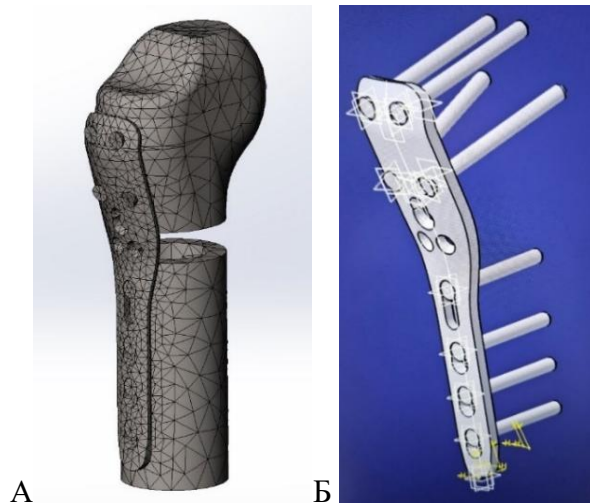
Рисунок 5 – Моделирование накостного остеосинтеза в программно-аналитических комплексах: А – 3D-модель плечевой кости в условиях накостного остеосинтеза пластиной и винтами. Модель кости имеет зону дефекта, обозначающего оскольчатую метафизарную зону. Б – 3D-пространственная модель реконструктивной пластины с угловой стабильностью винтов
