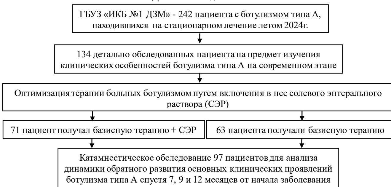
Рисунок 1 – Дизайн исследования
